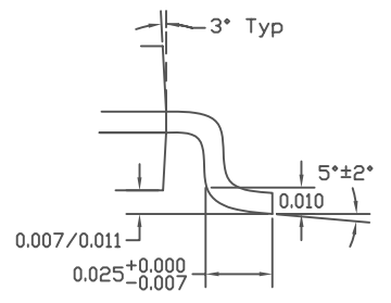
DETAIL A-A
